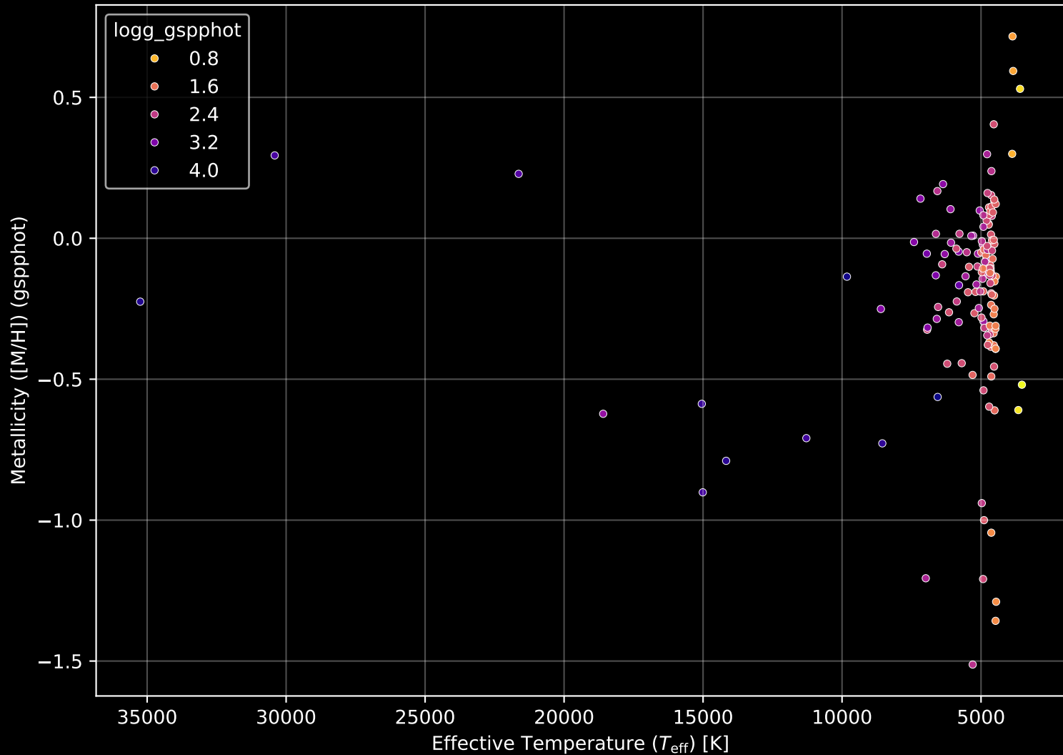
APOGEE DR17 Field: [Per_E] Stellar Population Parameters (n= 147)
